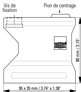
Trou de montage ouvert
